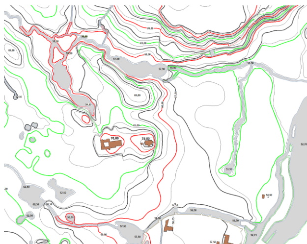
Rys. 28. Odtworzone ukształtowanie terenu wzgórza Świętego Wojciecha z XVIII w. [oprac. własne]
