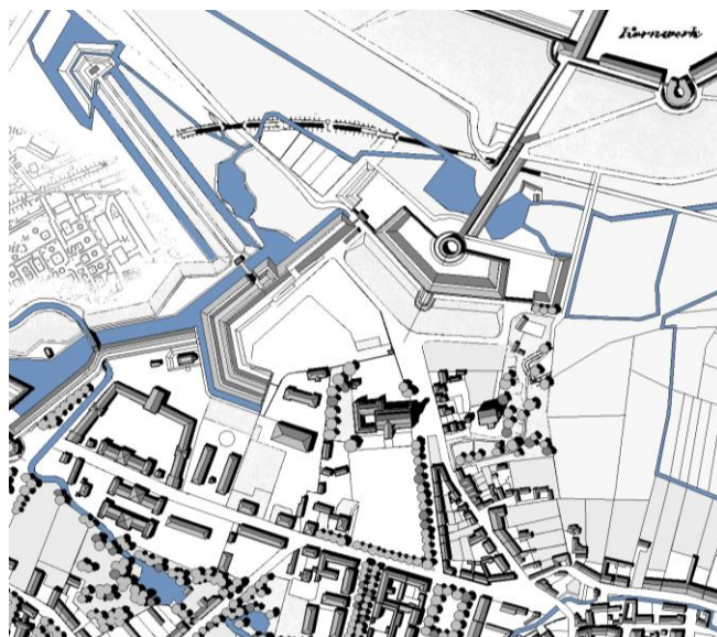
Rys. 5. Plan przedstawiający obszar Świętego Wojciecha w XIX w. z widocznym układem fortyfikacji i zabudowy Twierdzy Poznań oraz przekształconym układem wodnym [oprac. własne]
