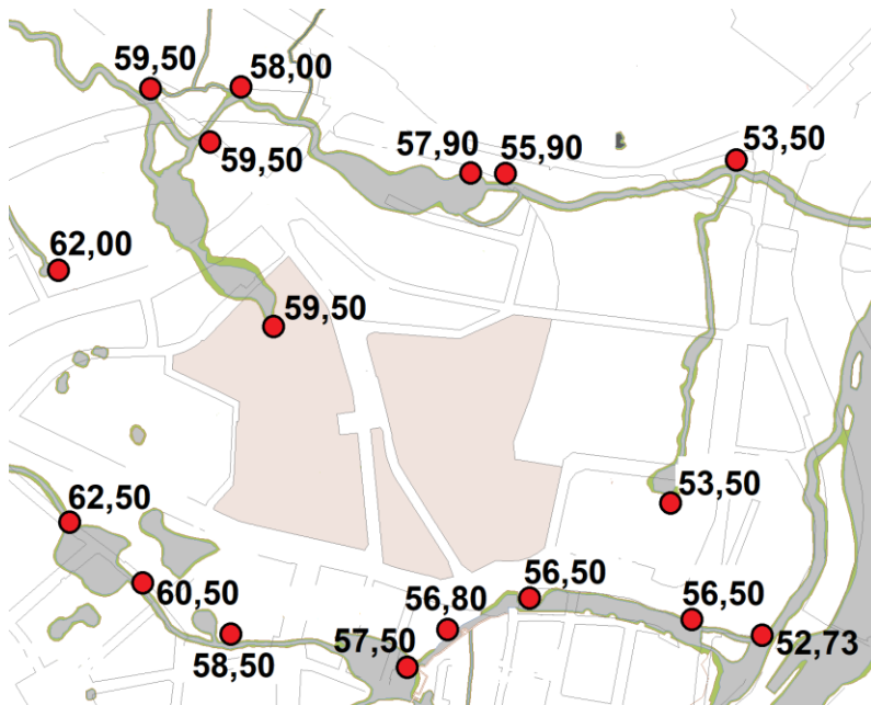
Rys. 24. Odtworzony układ wodny z XVIII w. wraz z jego rzędnymi wysokościowymi obszaru Świętego Wojciecha nałożony na współczesny układ kwartałów [oprac. własne]
